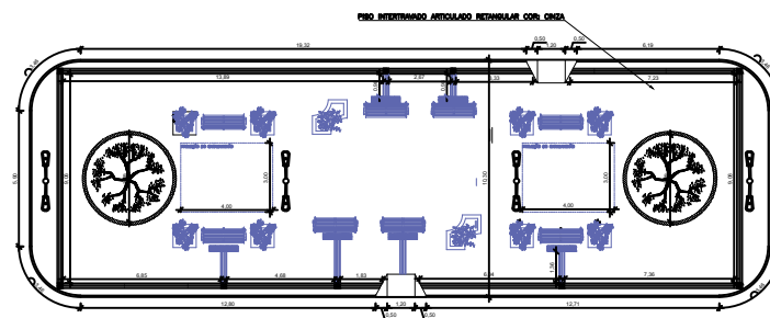
PLANTA DE AMPLIAÇÃO - PRAÇA DA EEF SANTA ADELAIDE (BITUPITÃ) PROJ. 1175 ÁREAS A SEREM CONSTRUÍDAS
