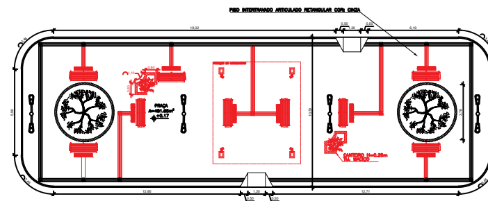
PLANTA DE DEMOLIÇÃO - PRAÇA DA EEF SANTA ADELAIDE (BITUPITÃ) PROJ. 1175 ÁREAS A SEREM DEMOLIDAS
