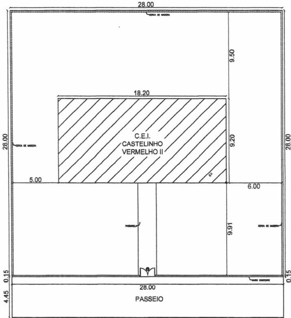
02 PLANTA BAIXA - EXISTENTE ESCALA - 1 : 100
