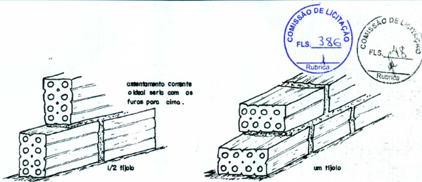
Figura 1 - Execução de alvenaria utilizando tijolos furados.
