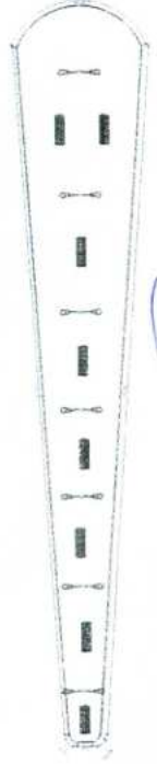
DETALHE BANCO DE MADEIRA ESC. 1/20
