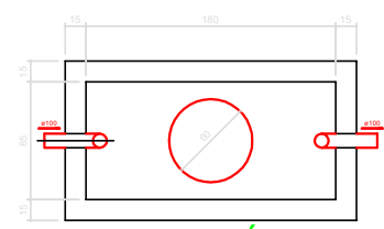
TANQUE SÉPTICO PLANTA BAIXA
