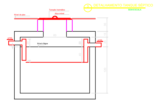
TANQUE SÉPTICO CORTE
