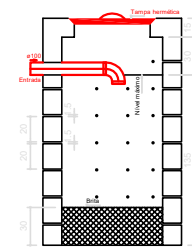
SUMIDOURO CORTE
