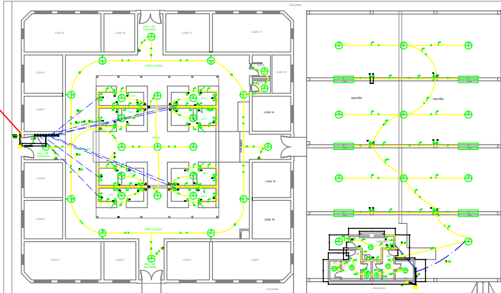
PLANTA BAIXA ELÉTRICA SEM ESCALA
