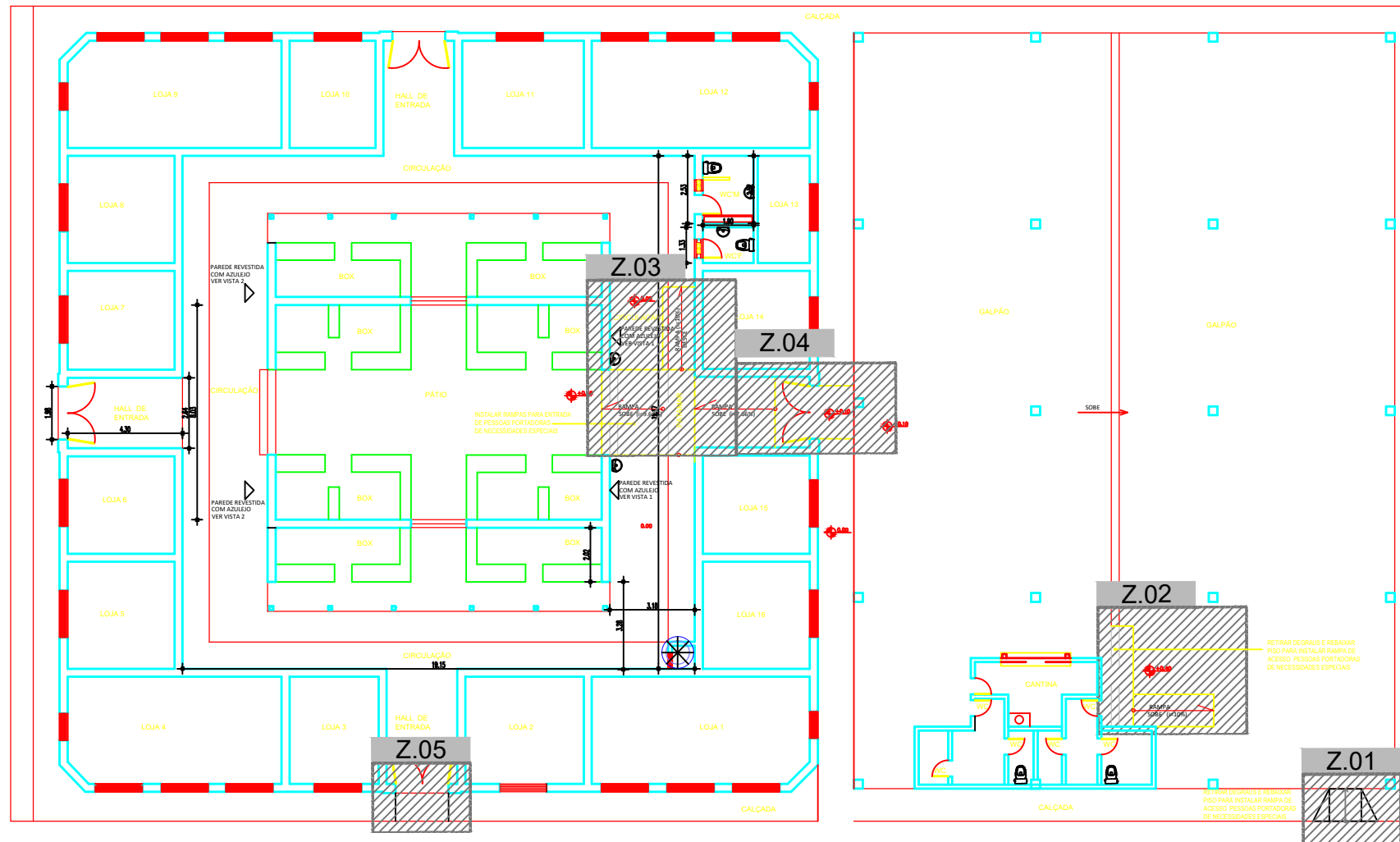
1 PLANTA BAIXA – GERAL ESCALA 1/100
