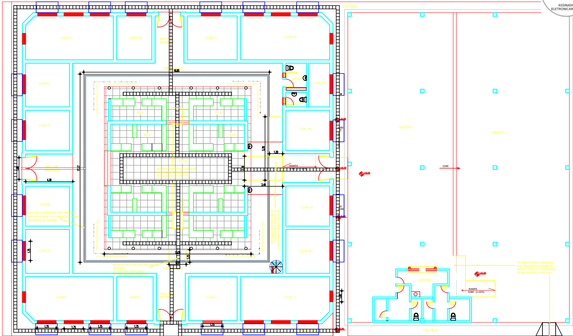
1 PLANTA BAIXA - LAYOUT GERAL ESCALA 1/100
