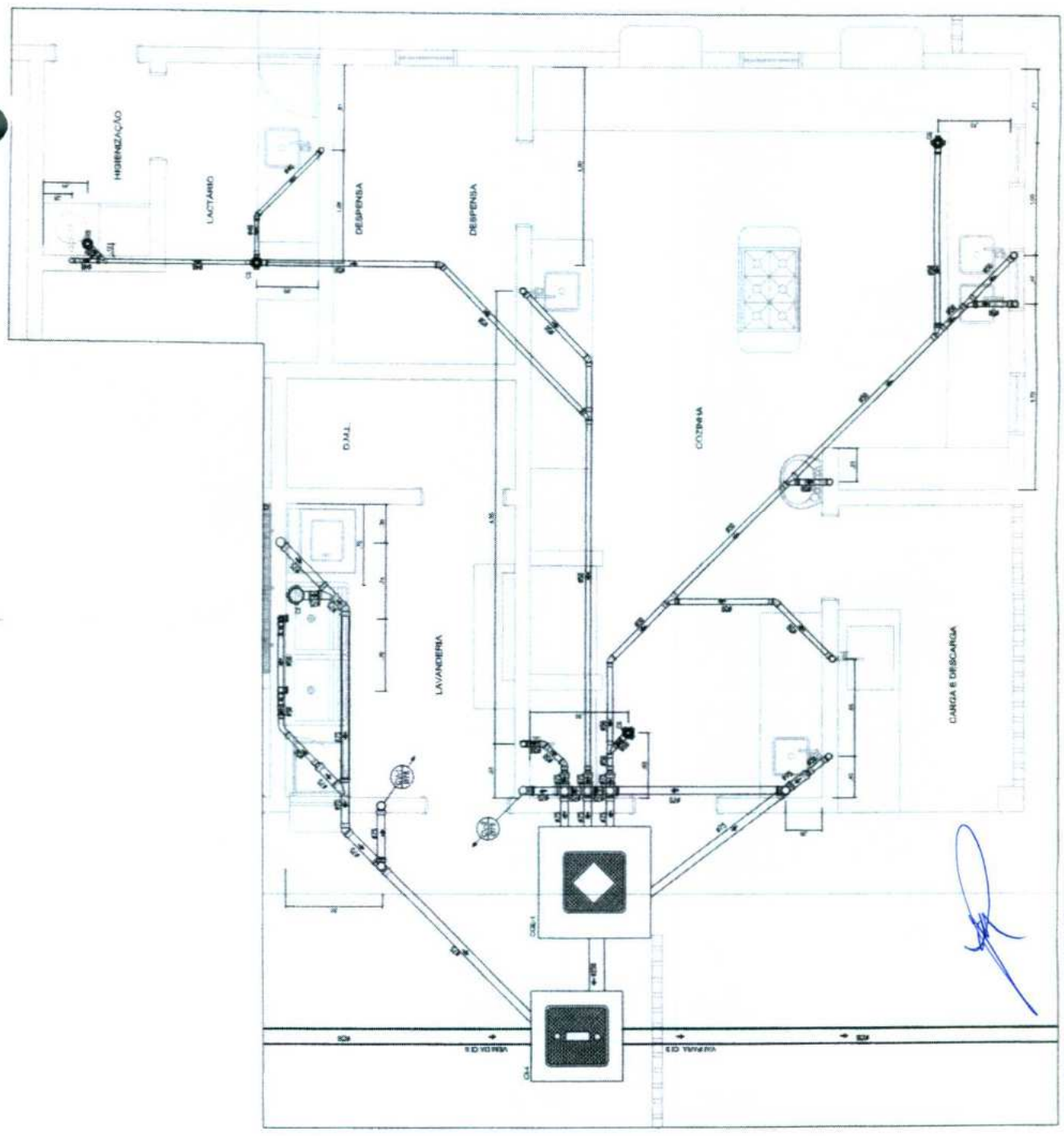
1 - LAVANDERIA, COZINHA, LACTÁRIO, HIGIENIZAÇÃO MAY 2016
